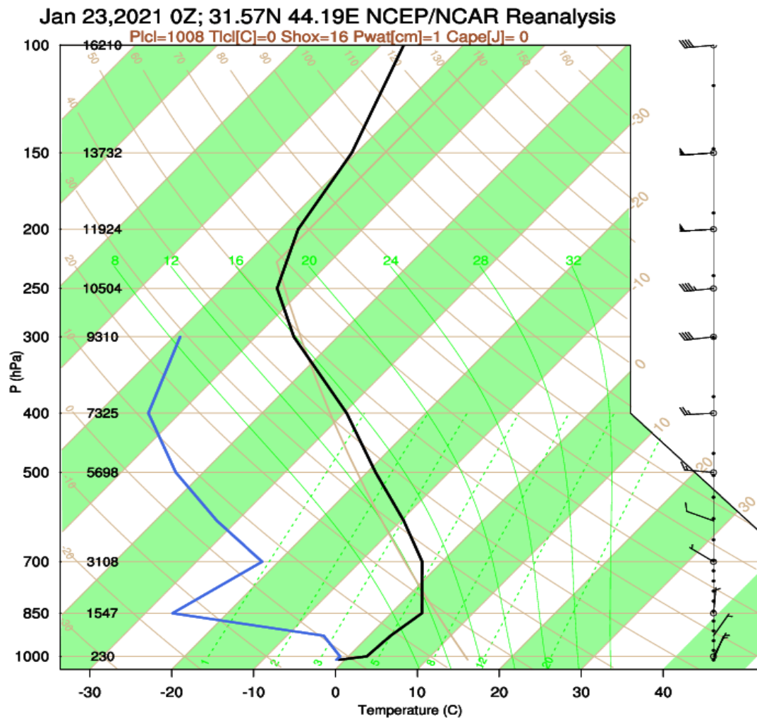
شكل (٤) مخطط Skew-T يوم (٢٠٢١/١/٢٣) لمحطة النجف
